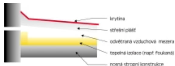
Zateplování dvouplášťové střechy s odvětranou mezerou. © EkoWATT
