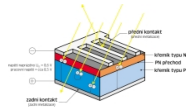
Princip činnosti solárního článku. © EkoWATT
