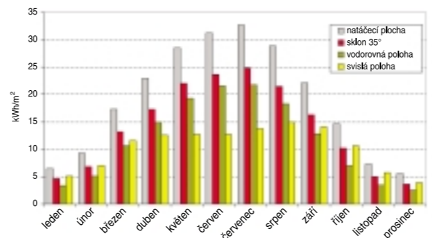
Odhad produkce fotovoltaického panelu. Zdroj: EkoWATT
