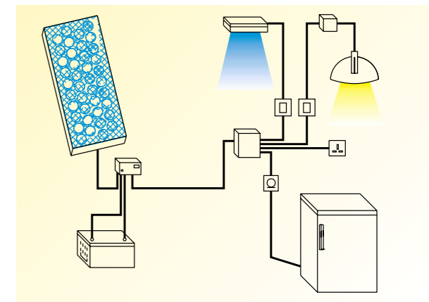
Schéma zapojení ostrovního systému. © EkoWATT
